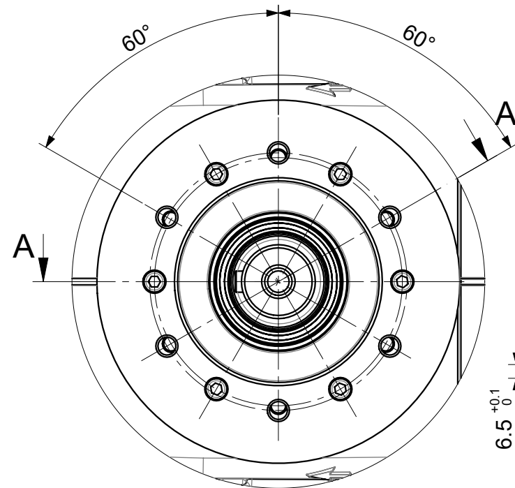
Dett."X": Scala 1:2,5
